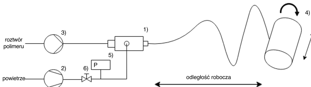
Rys. 1 Schemat stanowiska do produkcji nanowłóknin metodą rozdmuchu roztworu polimeru: 1) układ koncentrycznych dysz, 2) pompa powietrza, 3) pompa infuzyjna, 4) kolektor, 5) manometr, 6) zawór redukcyjny z osuszaczem powietrza.
